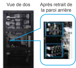
La conception de bornes fixes symétriques empêche tout problème de courbure des câbles afin de renforcer la fiabilité des câbles
